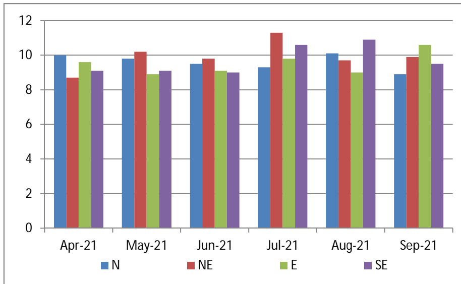
SO2
